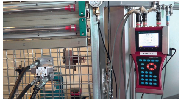
Um die Teilungsgenauigkeit des Volumenstroms zu erhöhen, kann zusätzlich ein Stromregelventil eingesetzt werden. Bild: fluid
