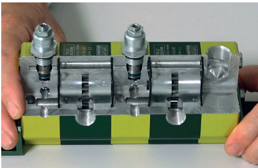
Ein Zahnradmengenteiler teilt das Öl durch kleine Zahnräder in gleichgroße Mengen auf und schickt es weiter in den Zylinder. Bild: fluid
