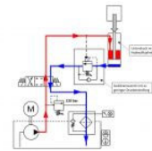
(files/upload/post/flu/2017/08/174638/hydraulikplan-zum-presseartikel-senkbremsventil-04-08-2017.jpg) Ölfluss bei negativer Last mit zu gering eingestelltem Senkbremsventil. Bild IHA
