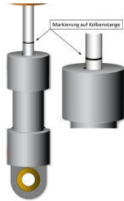
(files/upload/post/flu/2017/08/174638/zyinder-mit-stangenmarkierung-peter-poppick-27-06-2017.jpg) Markierung auf Kolbenstange mittels Permanentmarker. Bild: IHA
